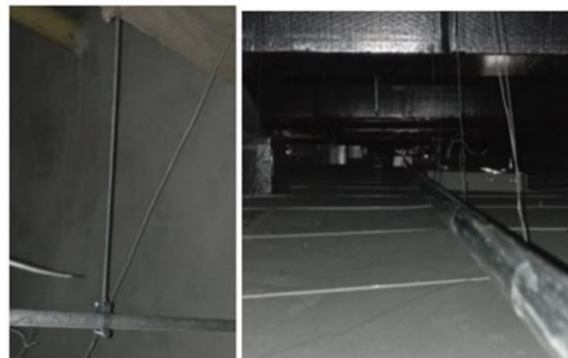
Figura 61- Plano instalación sensor de humo
