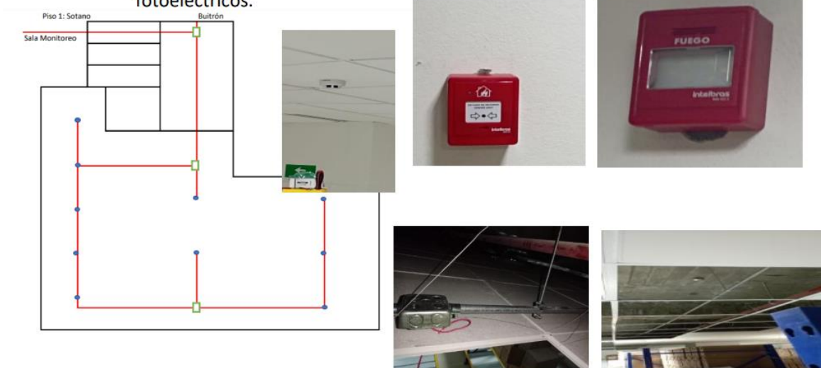
Figura 59.1- Plano instalación sensor de humo
