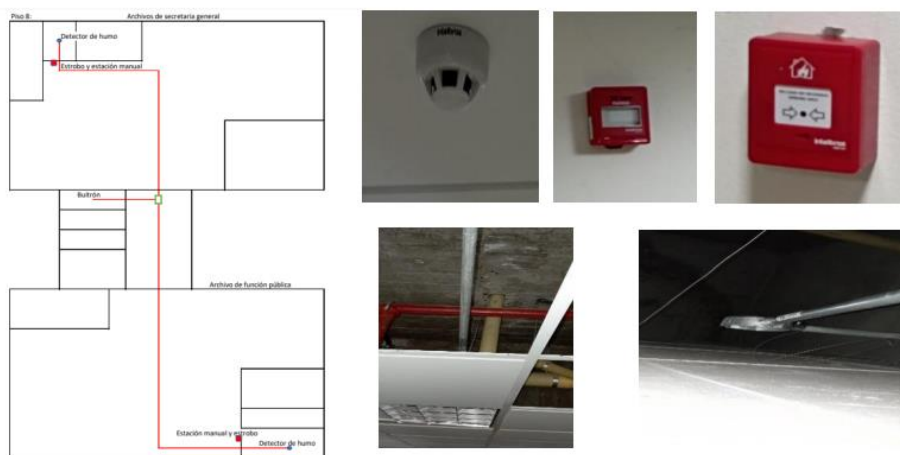
Figura 55- Plano instalación sensor de humo
