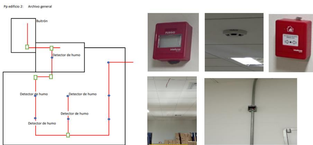
Figura 59- Plano instalación sensor de humo
