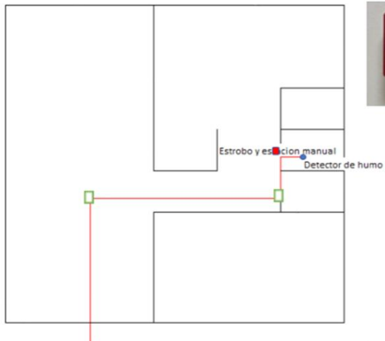
Figura 61- Plano instalación sensor de humo
