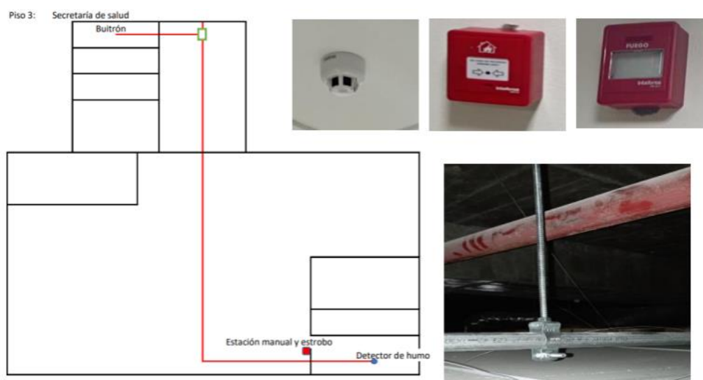
Figura 58- Plano instalación sensor de humo
