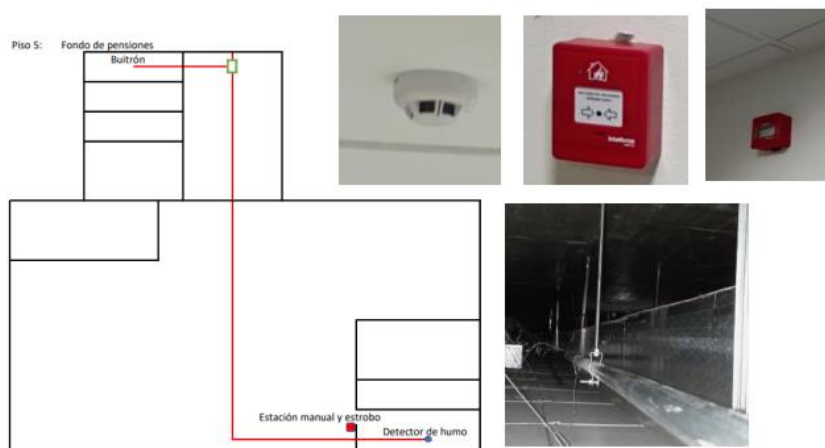
Figura 56- Plano instalación sensor de humo
